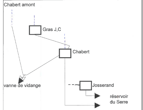
Vanne vidange (schéma de principe)
